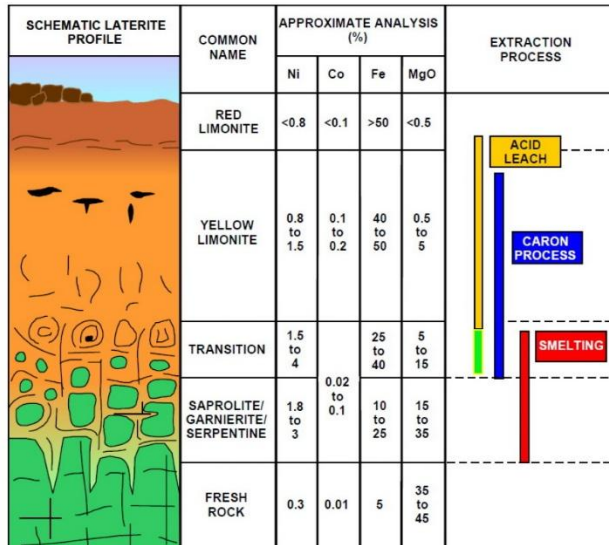
Gambar 27. Profil Nikel laterit (Sumber: Waheed, 2008 dalam Kyle, 2010)
